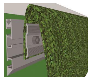
Klemmung mit Alu-Profil bei starker Last
